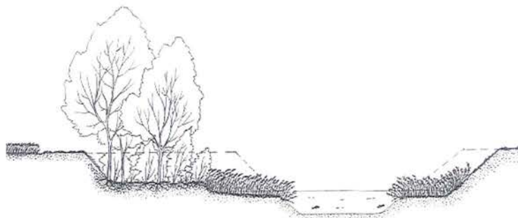
Figura 2 Ampliamento sezione canale (disegno Massimo Milandri)
