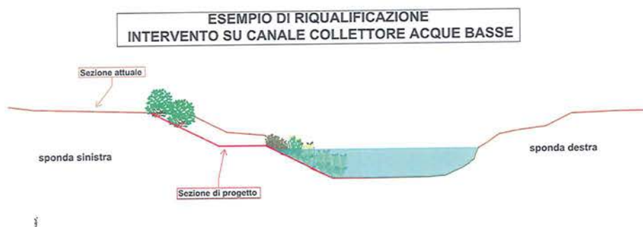
Figura 3 - Esempio di riqualificazione (disegno Consorzio di Bonifica dell'Emilia Centrale)
